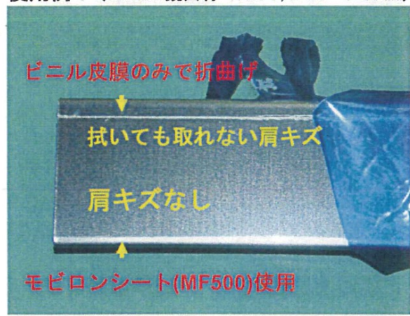
使用例1 (SUS430 鏡面材 1.2t P/D=88° V=10mm)
