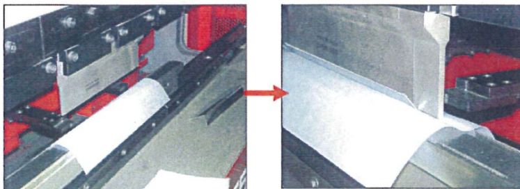
使用例1 (SUS430 鏡面材 1.2t P/D=88° V=10mm)
