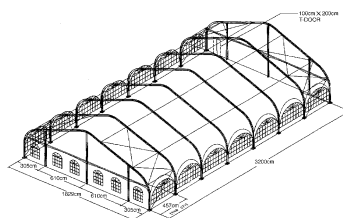
参考例 7スパンの場合 ●全体サイズ：W18m×D32m×H6.5m
