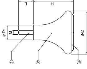
材質 ①ボルト：鋼(3価クロメート) ②本体：ABS ③底脚：ABS
